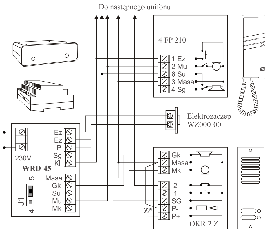
Schemat 2 - system 5 przewodowy - unifon TESLA 4 FP 210
